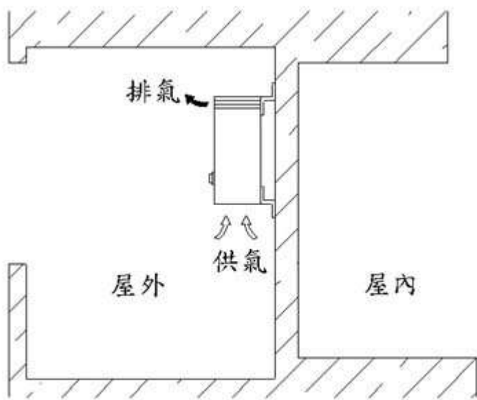
〈圖 1〉 室外型熱水器安裝圖
